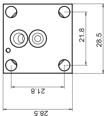
C-seal尺寸图
