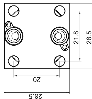
W-seal尺寸图
