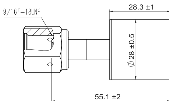
1/4FVCR尺寸图
