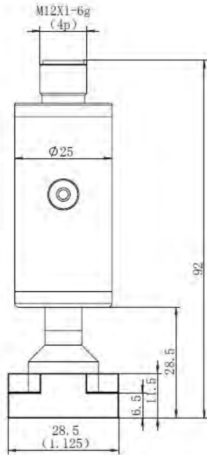
C-Seal(1.125")
